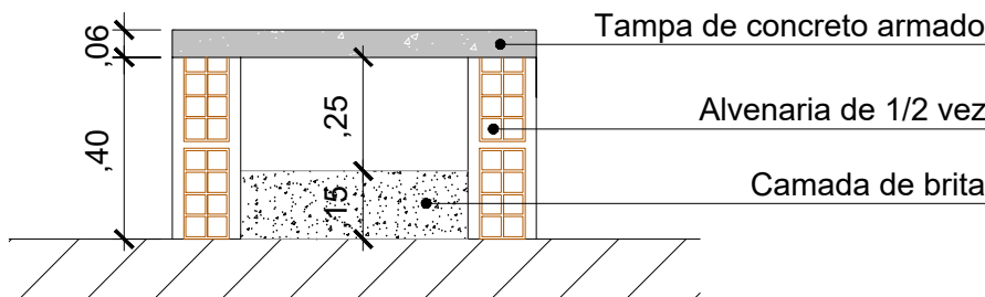
CORTE AA
