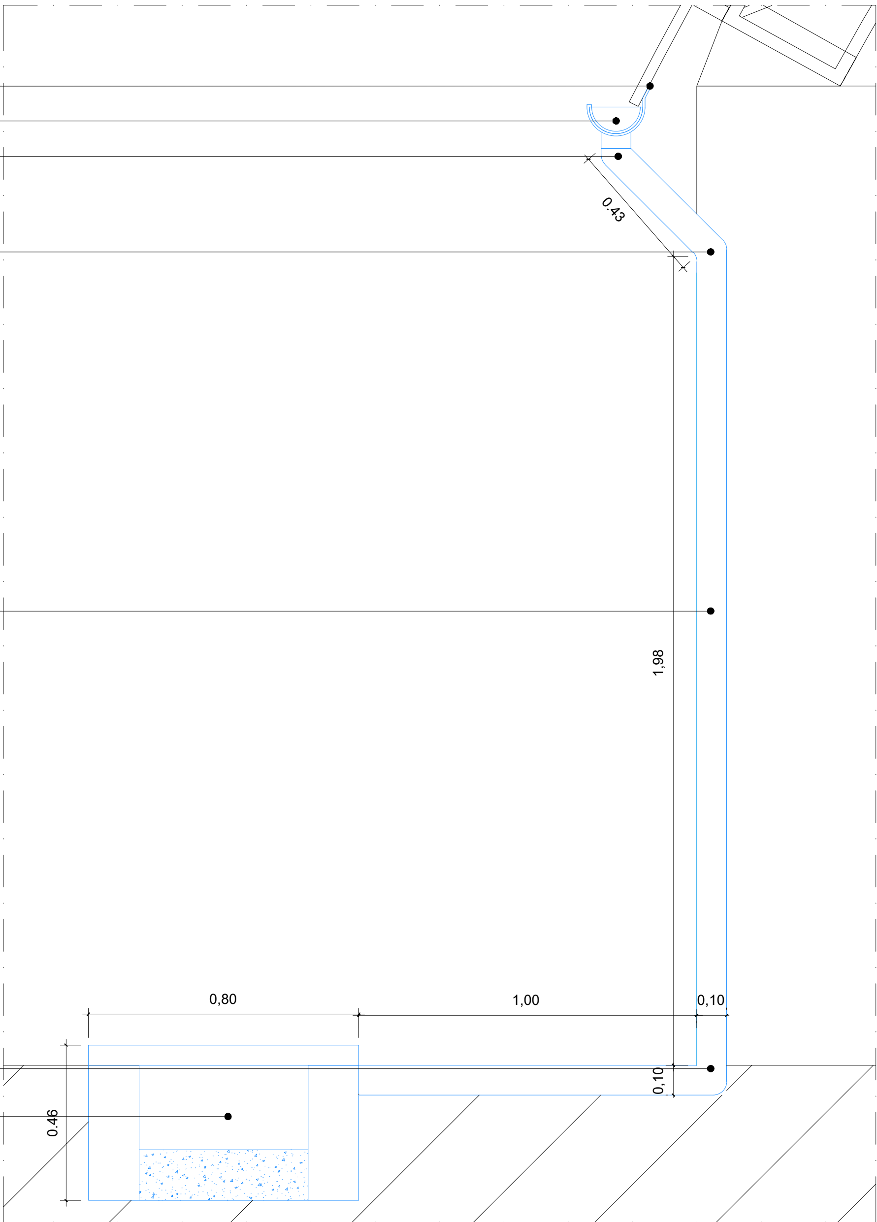
Detalhe 01
