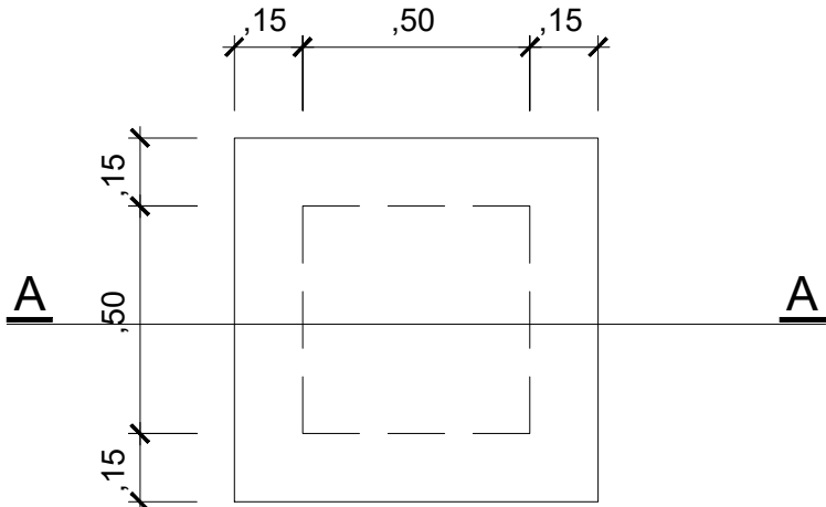
PLANTA BAIXA
